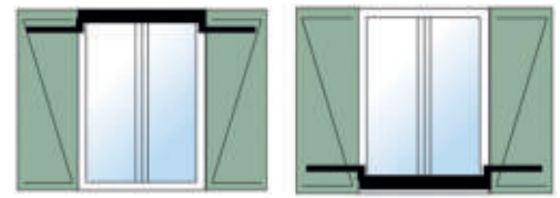
Pose sous linteau
