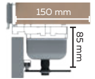
Coupe précadre et capot
