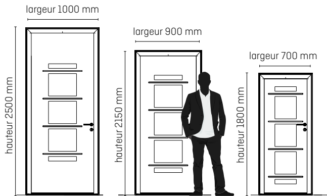
VOLT Dimensions MINI ou MAXI : 100% des modèles Zilten réalisables en SUR-MESURE (hauteur 2500 mm sans imposte sur certains modèles).
