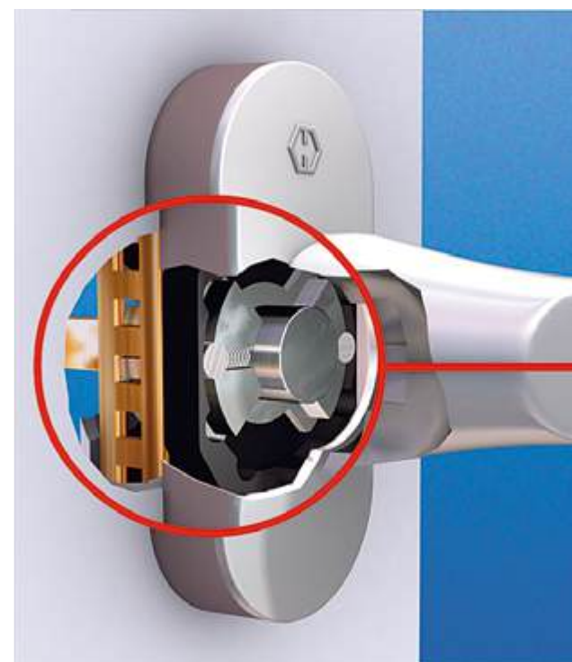
POIGNÉE SECUSTIK® INCROCHETABLE
