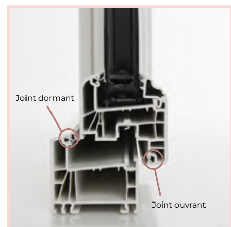
2 JOINTS D'ISOLATION
