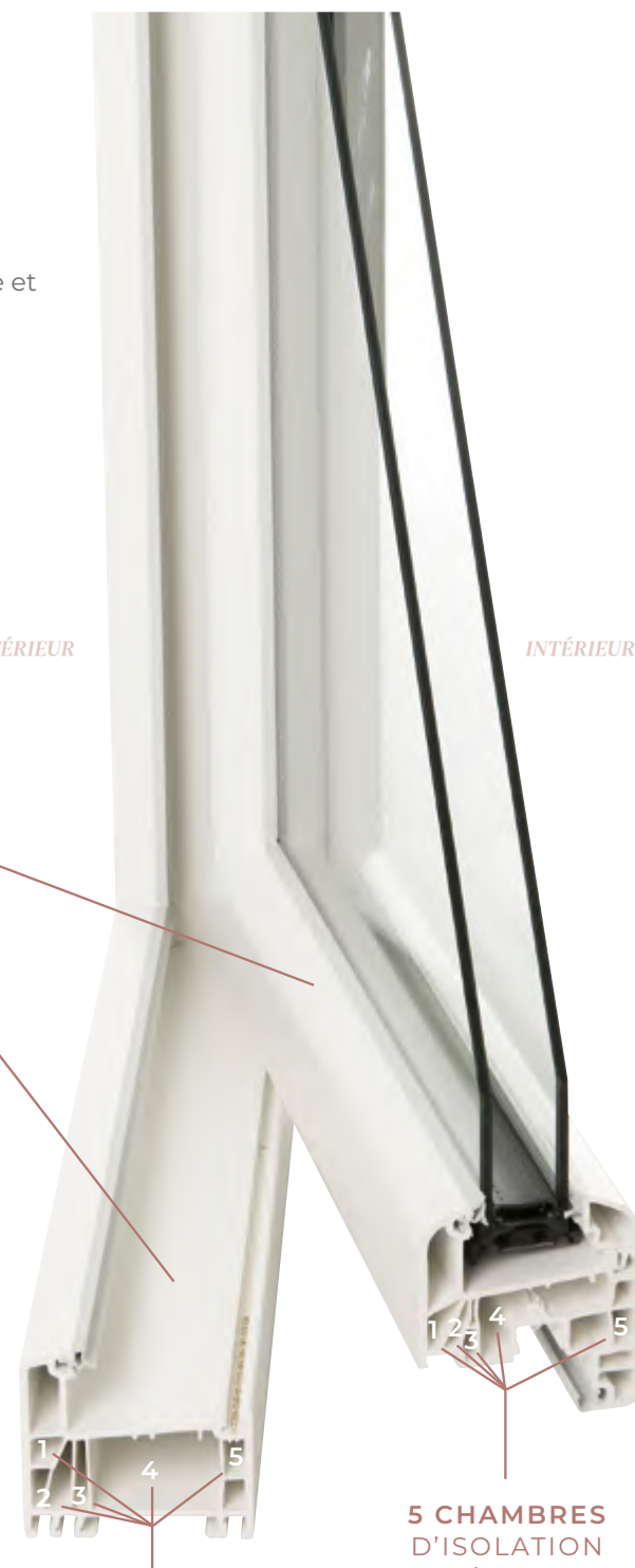
5 CHAMBRES D'ISOLATION SUR LE DORMANT
